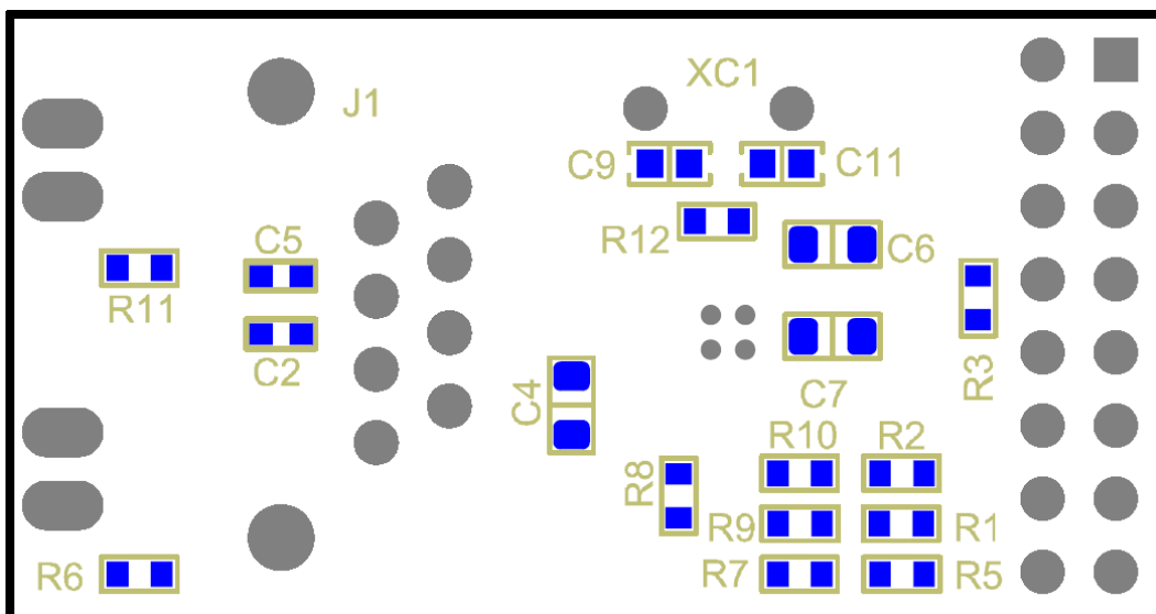
Плата, нижняя сторона
