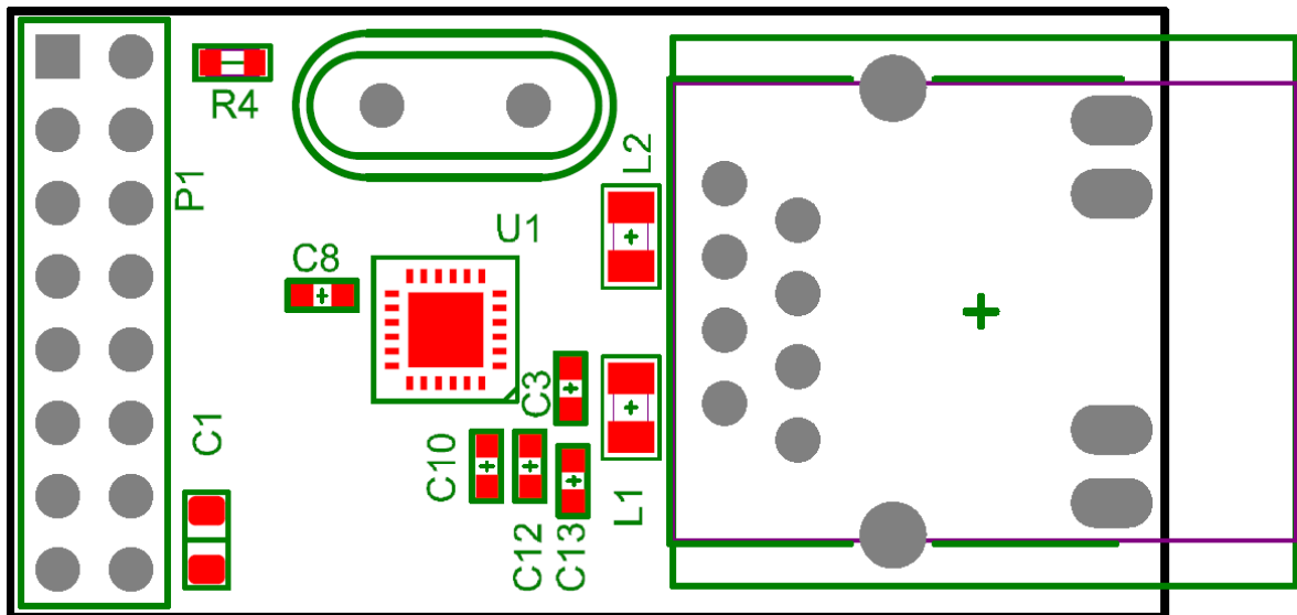
Плата, верхняя сторона
