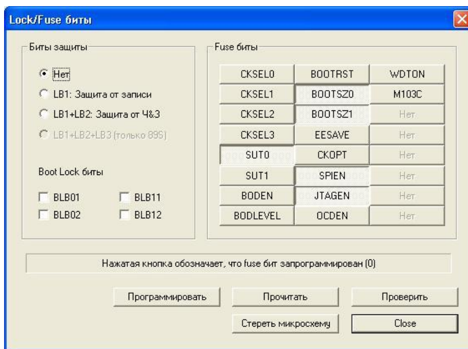
Рисунок 1. Предустановки микросхемы ATmega128A
